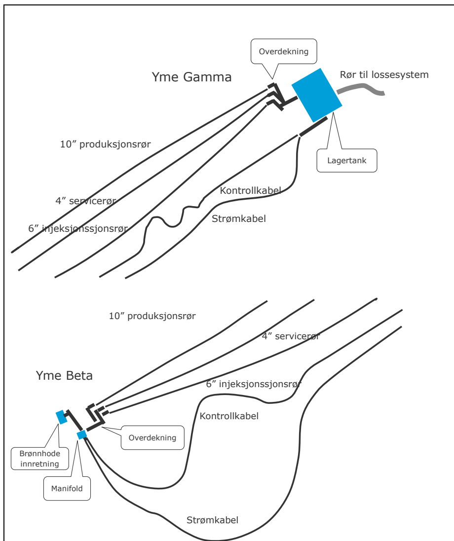
Figur 2-5. Skisse over plassering av innretninger, rørledninger og annen infrastruktur.
