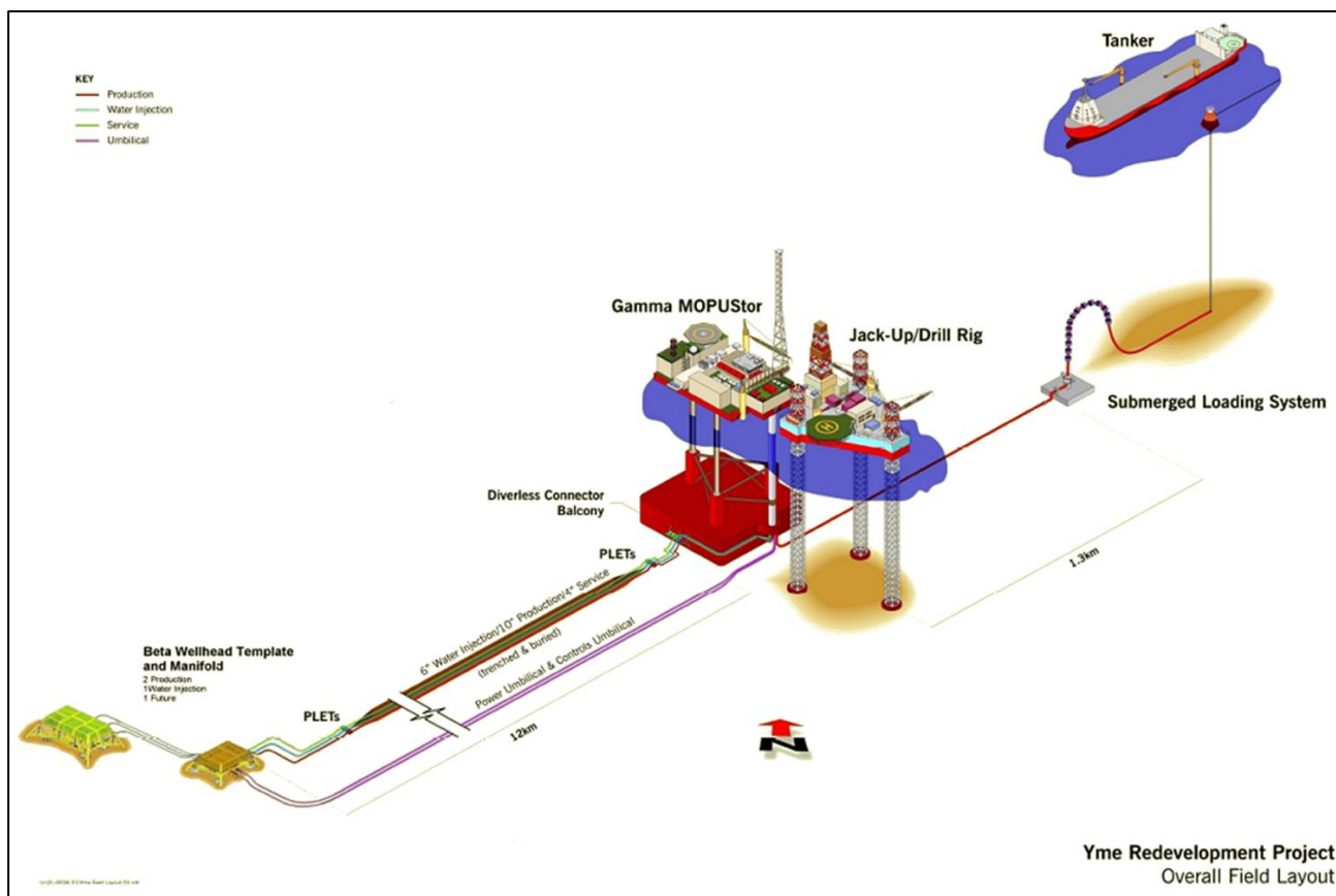
Figur 2-2. Innretninger på Yme-feltet. Sjøbunnslinnetningene inngår i denne konsekvensutredningen (lagertank under overbygningen, rørledninger og havbunnsinstallasjoner). I figuren vises også tankskip for oljeeksport, midlertidig oppjekkbar borerigg og overbygning som står på lagertanken på bunn, men disse installasjonene inngår ikke i KU.
