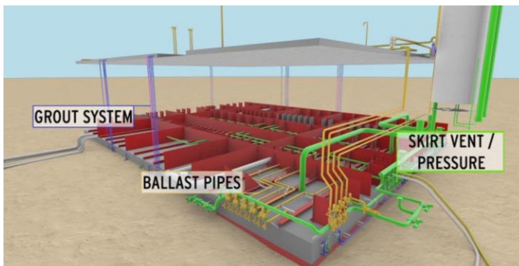
Figur 2-4. Skisse av lagertanken på sjøbunnen og midlertidig bruk av borerigg. Nederst er en illustrasjon av innvendig inndeling i tanken og tilhørende rørsystem.
